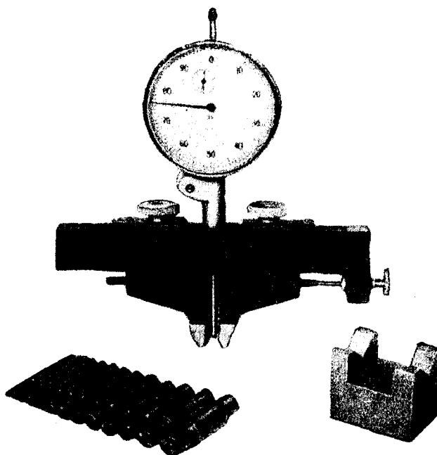
Зубомер тангенциальный, типа ЗТ
